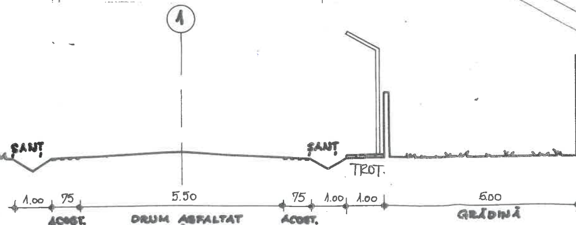
PROFIL TRANSVERSAL SC. 1:100
